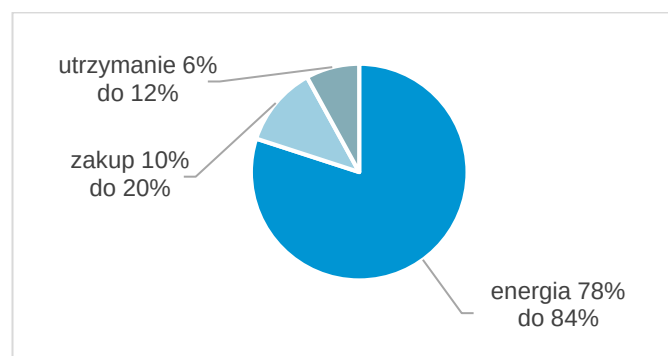
Rysunek 8 Udziały poszczególnych kosztów w LCC dla instalacji sprężonego powietrza
