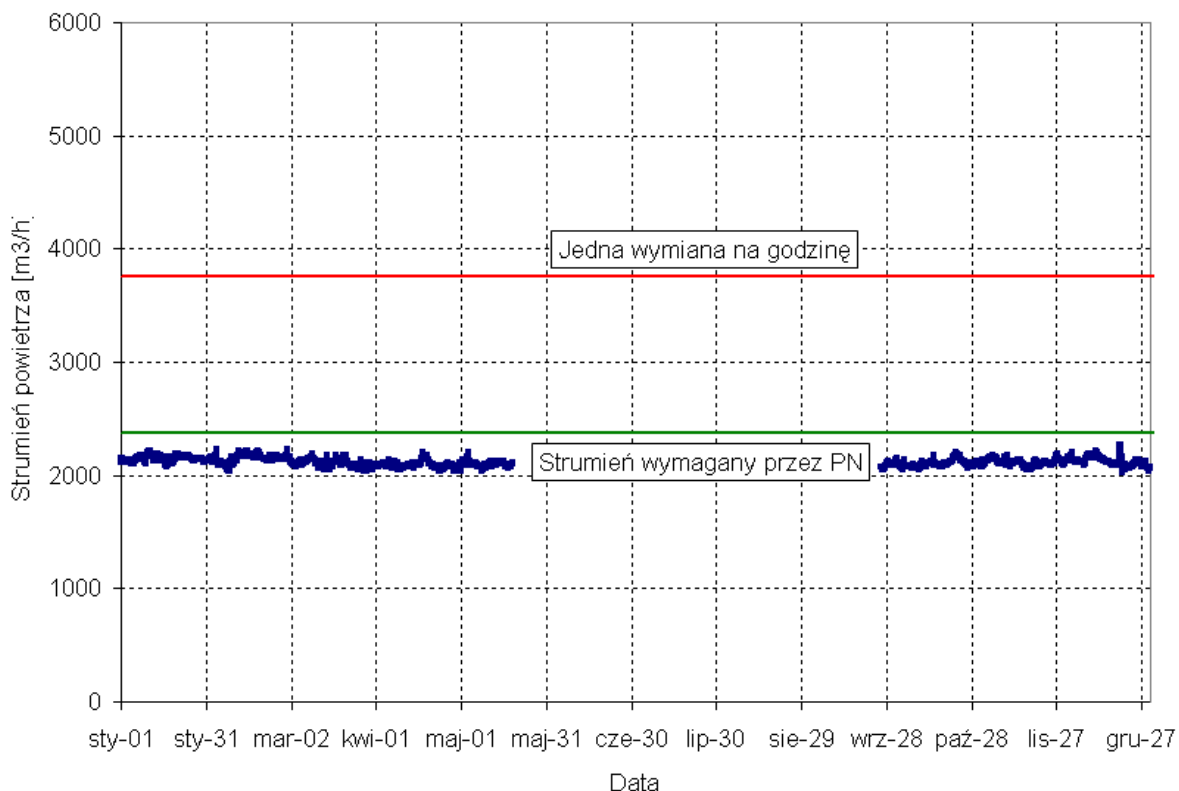
Rys. 49. Przebieg zmienności strumienia powietrza dla mieszkań.
