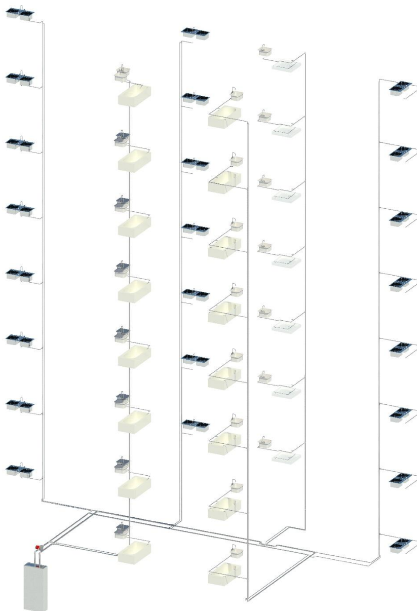
Rys. 21. Aksonometria instalacji c.w.u. i instalacji cyrkulacyjnej.
