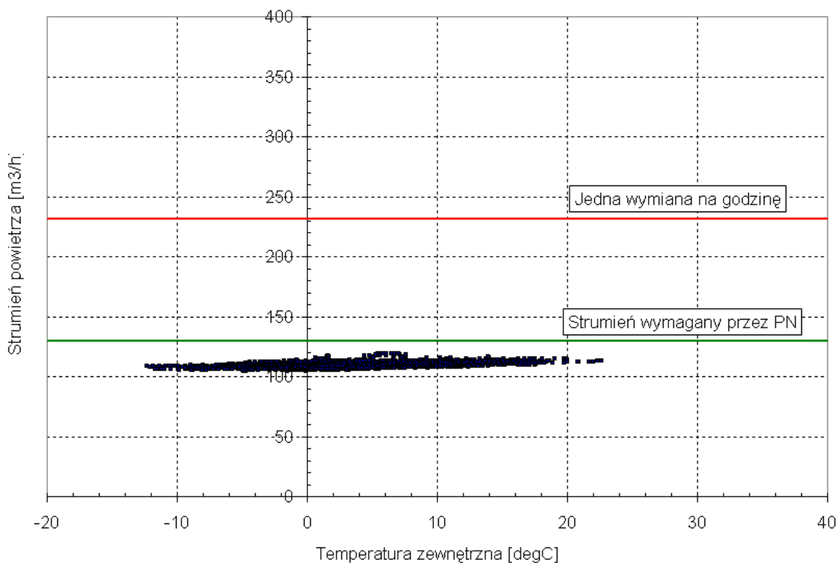
Rys. 56. Zależność strumienia powietrza dla mieszkania M3 na piątym piętrze od temperatury powietrza zewnętrznego.
