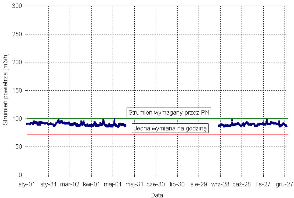
Rys. 57. Przebieg zmienności strumienia powietrza dla mieszkania M1 na pierwszym piętrze.
