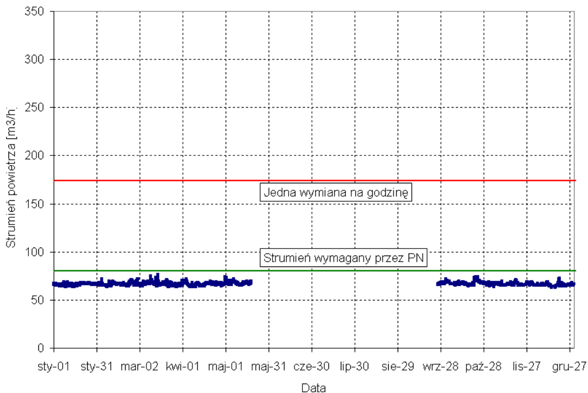
Rys. 53. Przebieg zmienności strumienia powietrza dla mieszkania M2 na piątym piętrze.
