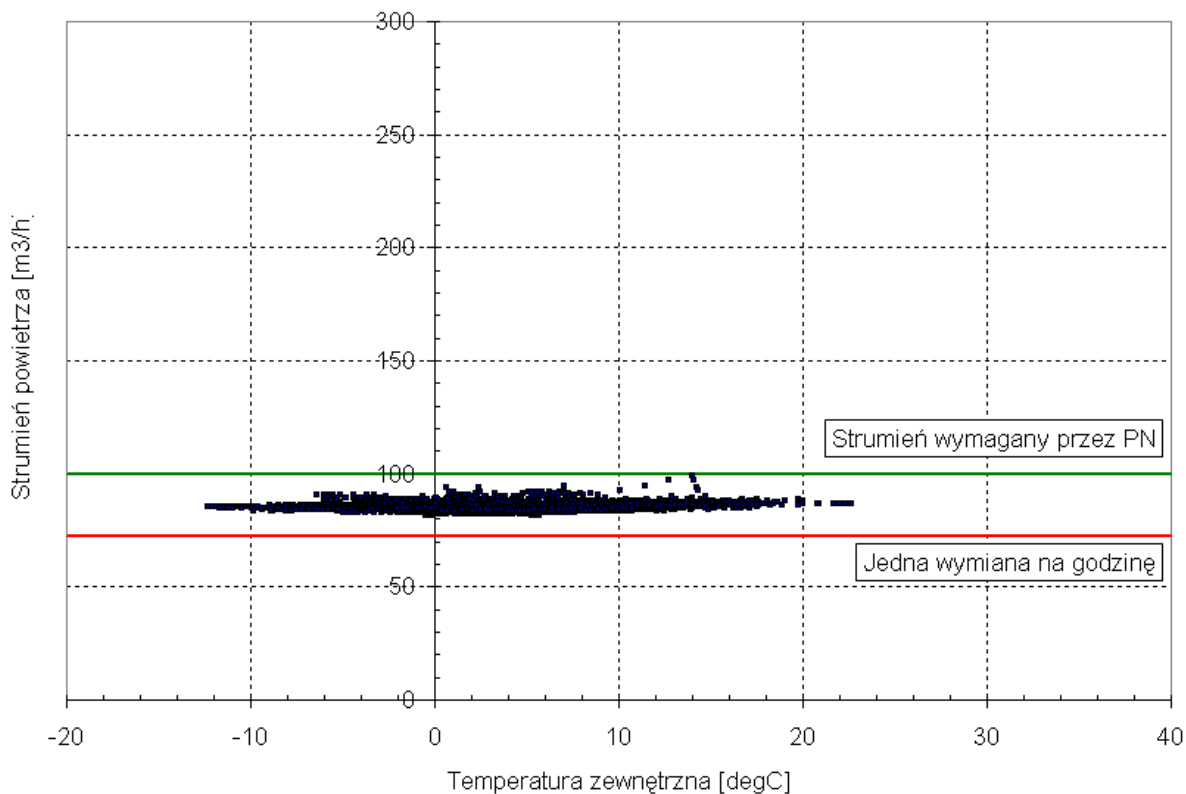
Rys. 52. Zależność strumienia powietrza dla mieszkania M1 na piątym piętrze od temperatury powietrza zewnętrznego.
