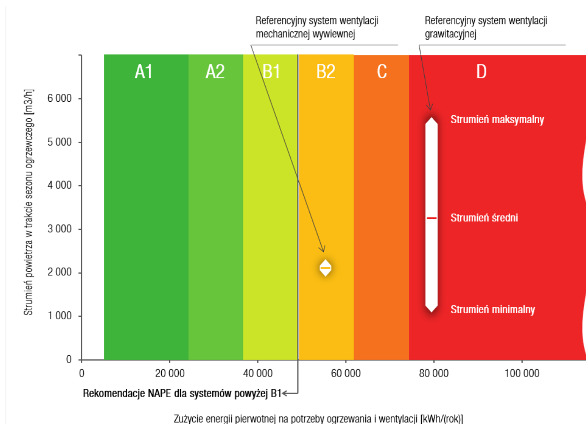
Rys. 73. Ilustracja kategorii efektywności energetycznej NAPE dla wielorodzinnego budynku referencyjnego NAPE wyposażonego w referencyjne systemy wentylacji grawitacyjnej i mechanicznej wywiewnej.
