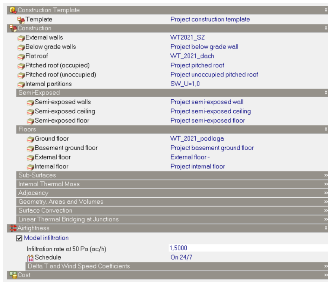
Rys. 65. Zakładka Construction do wprowadzenia danych dotyczących przegród budynku w programie DesignBuilder
